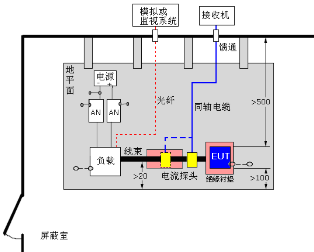
俯视图
