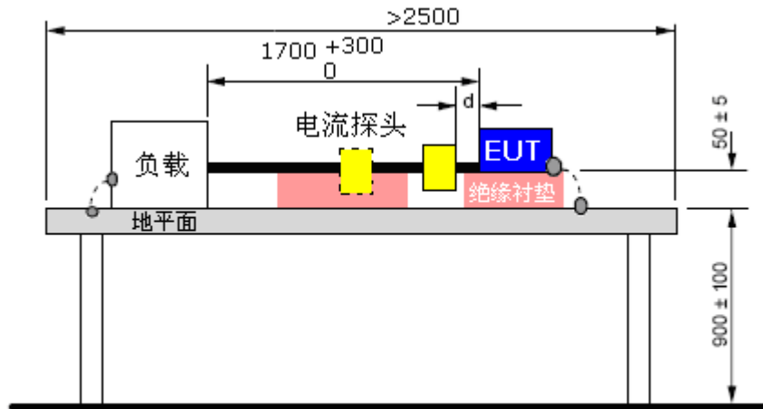
侧视图
